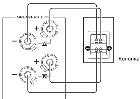
Задняя панель
